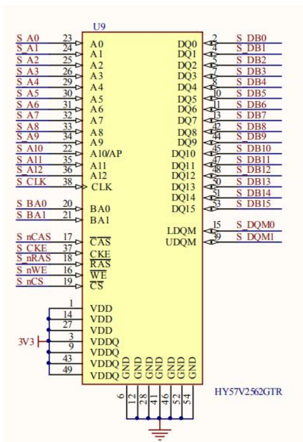
图 2-30SDRAM 原理图部分
